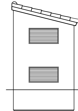
FACADE GAUCHE.
