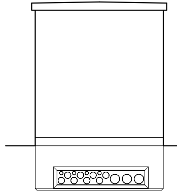
FAÇADE DROITE.
