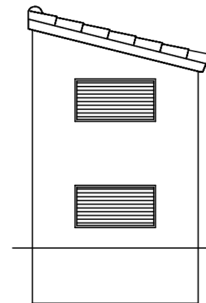
FACADE GAUCHE.
