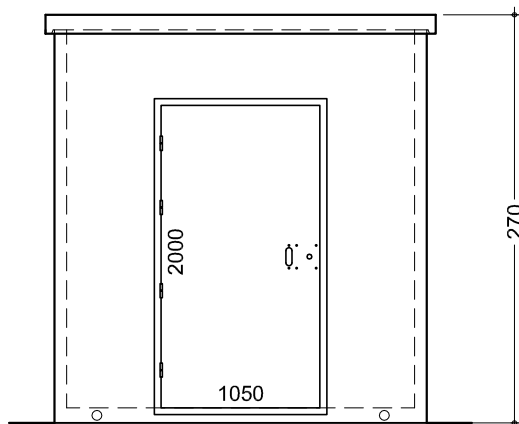
FAÇADE AVANT
